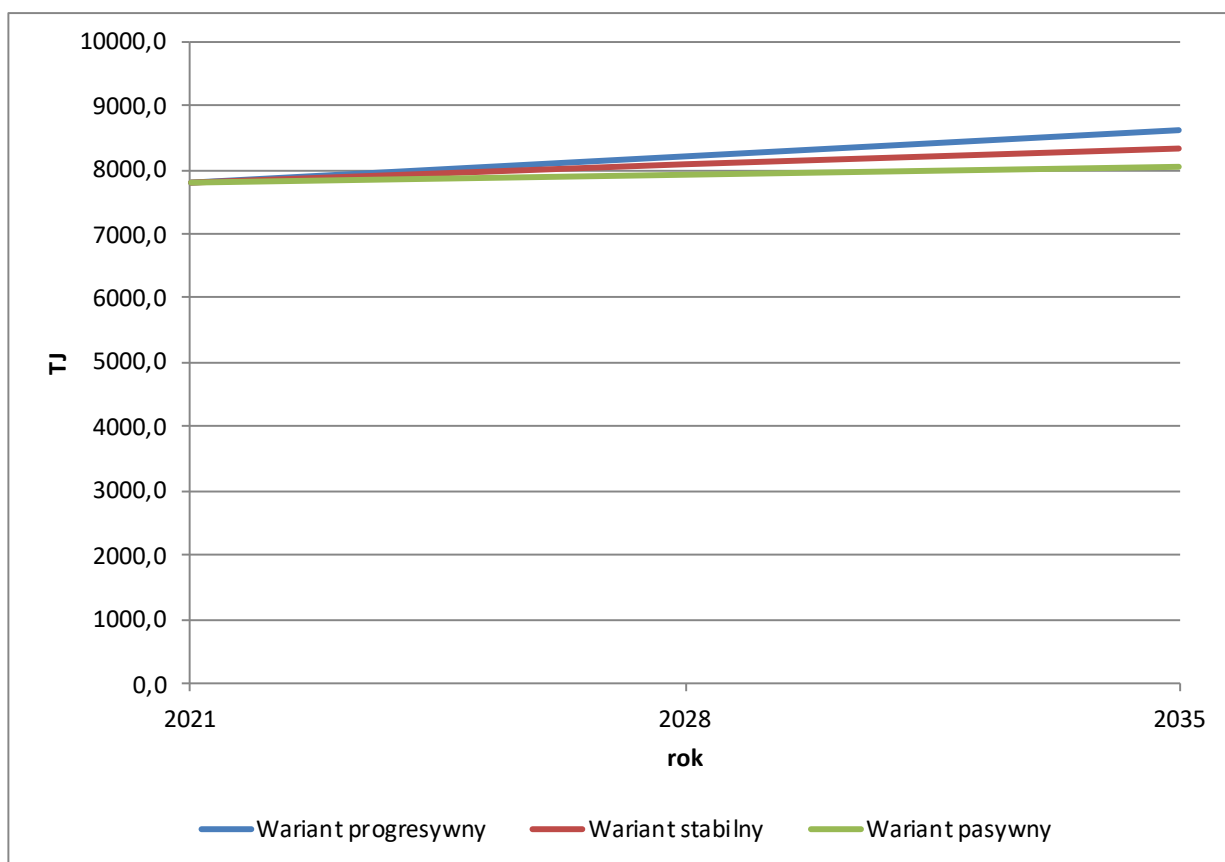
Rysunek 36. Prognozowana roczna zmiana zużycia ciepła do roku 2035.
