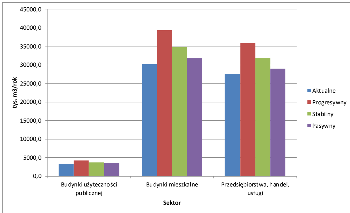
Rysunek 41. Szczegółowy bilans rocznego zapotrzebowania na paliwa gazowe na terenie powiatu cieszyńskiego.
