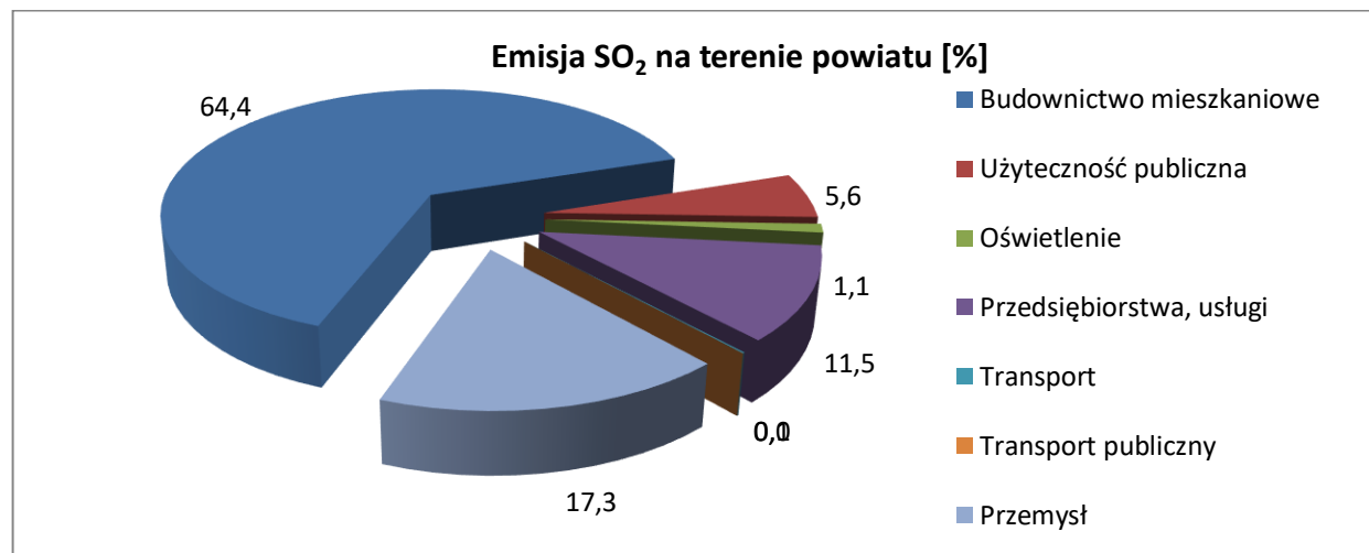
Rysunek 5. Emisja SO 2 w powiecie wg. sektorów.
