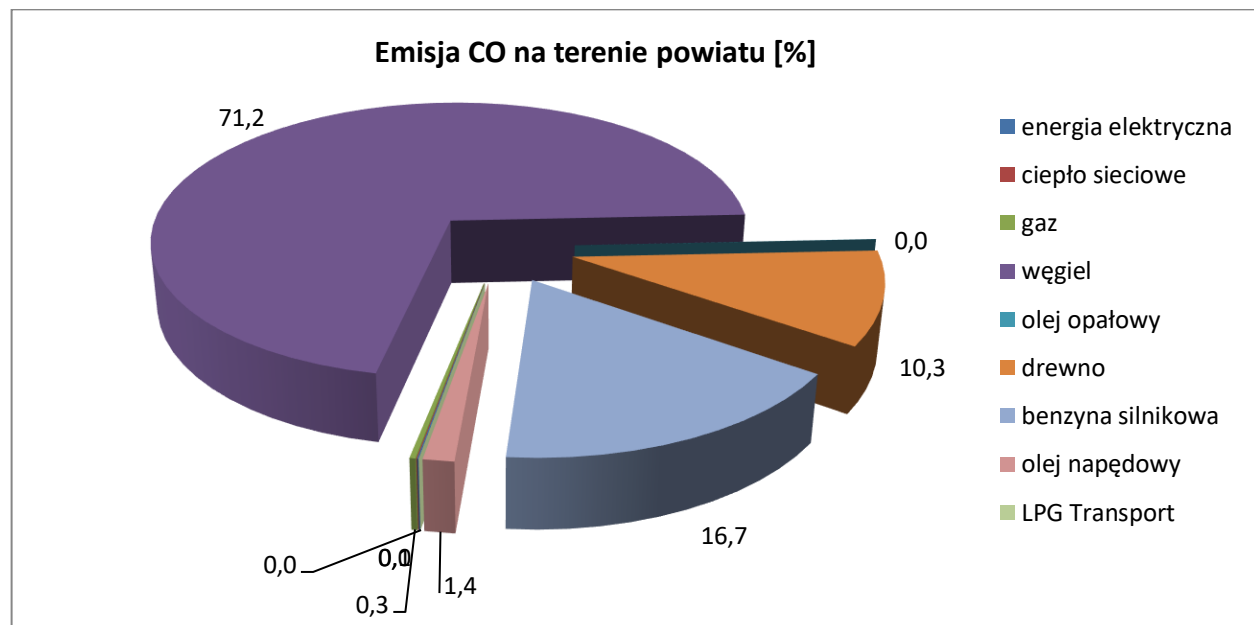
Rysunek 8. Emisja CO w powiecie wg. rodzajów paliw.
