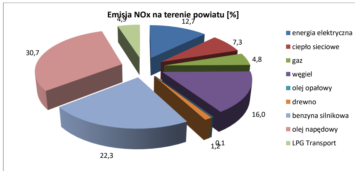
Rysunek 6. Emisja NOx w powiecie wg. rodzajów paliw.
