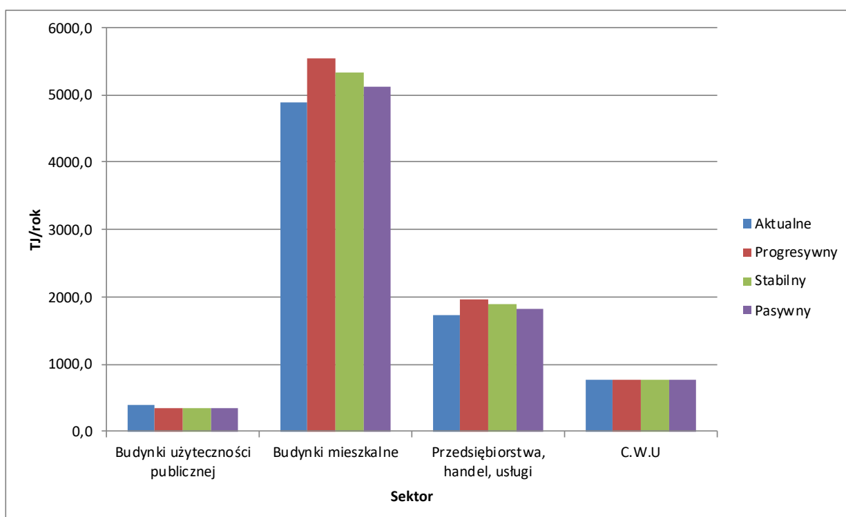
Rysunek 37. Szczegółowy bilans rocznego zapotrzebowania na ciepło na terenie powiatu cieszyńskiego.
