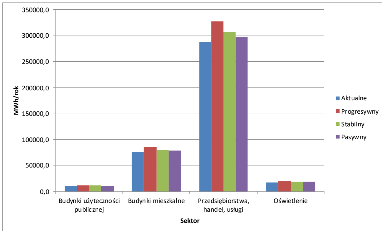
Rysunek 39. Szczegółowy bilans rocznego zapotrzebowania na energię elektryczną na terenie powiatu cieszyńskiego.
