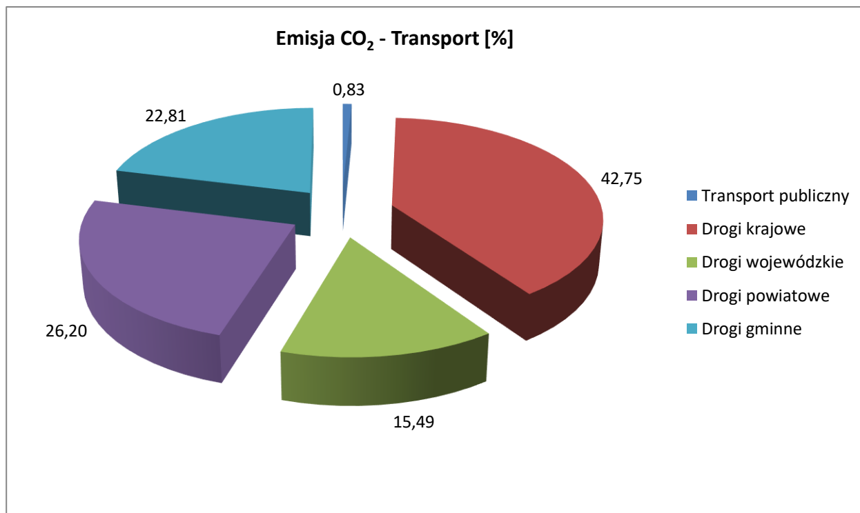
Rysunek 14. Emisja CO 2 wg. poszczególnych sektorów transportu.
