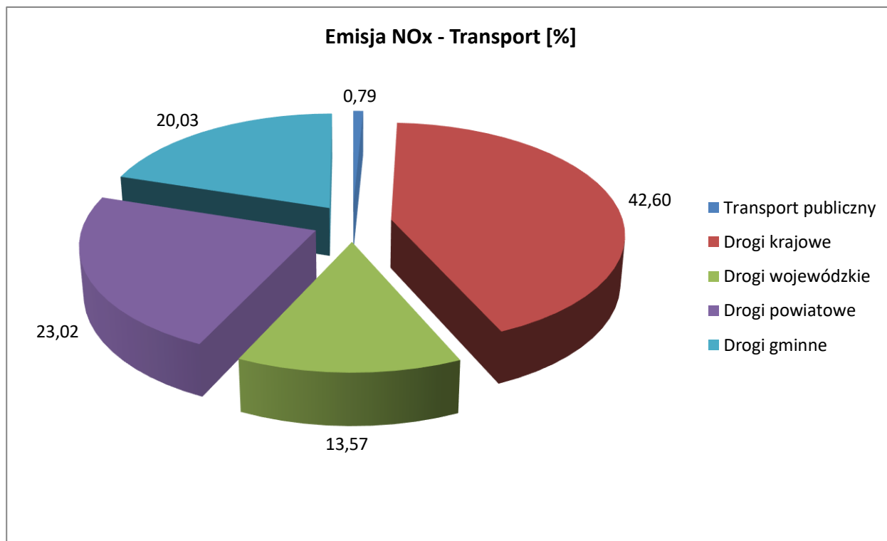
Rysunek 17. Emisja NOx wg. poszczególnych sektorów transportu.
