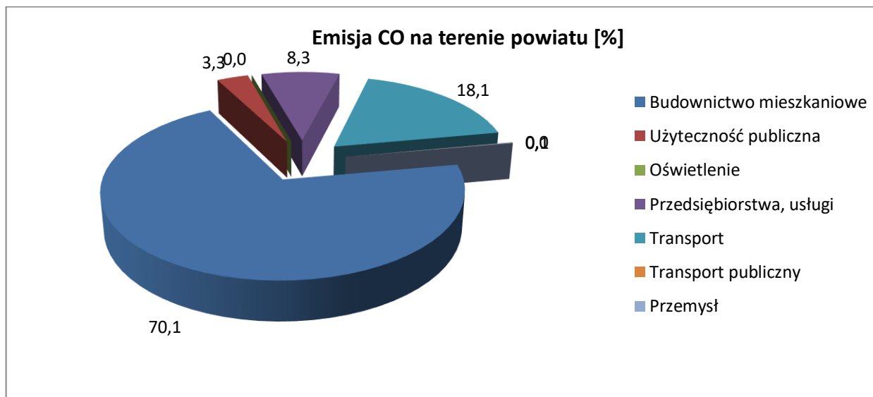
Rysunek 9. Emisja CO w powiecie wg. sektorów.
