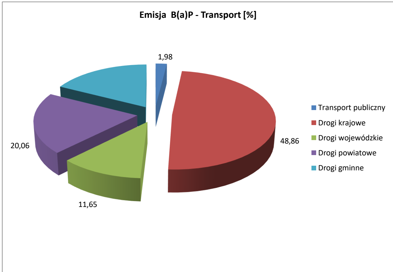
Rysunek 20. Emisja B(a)P wg. poszczególnych sektorów transportu.
