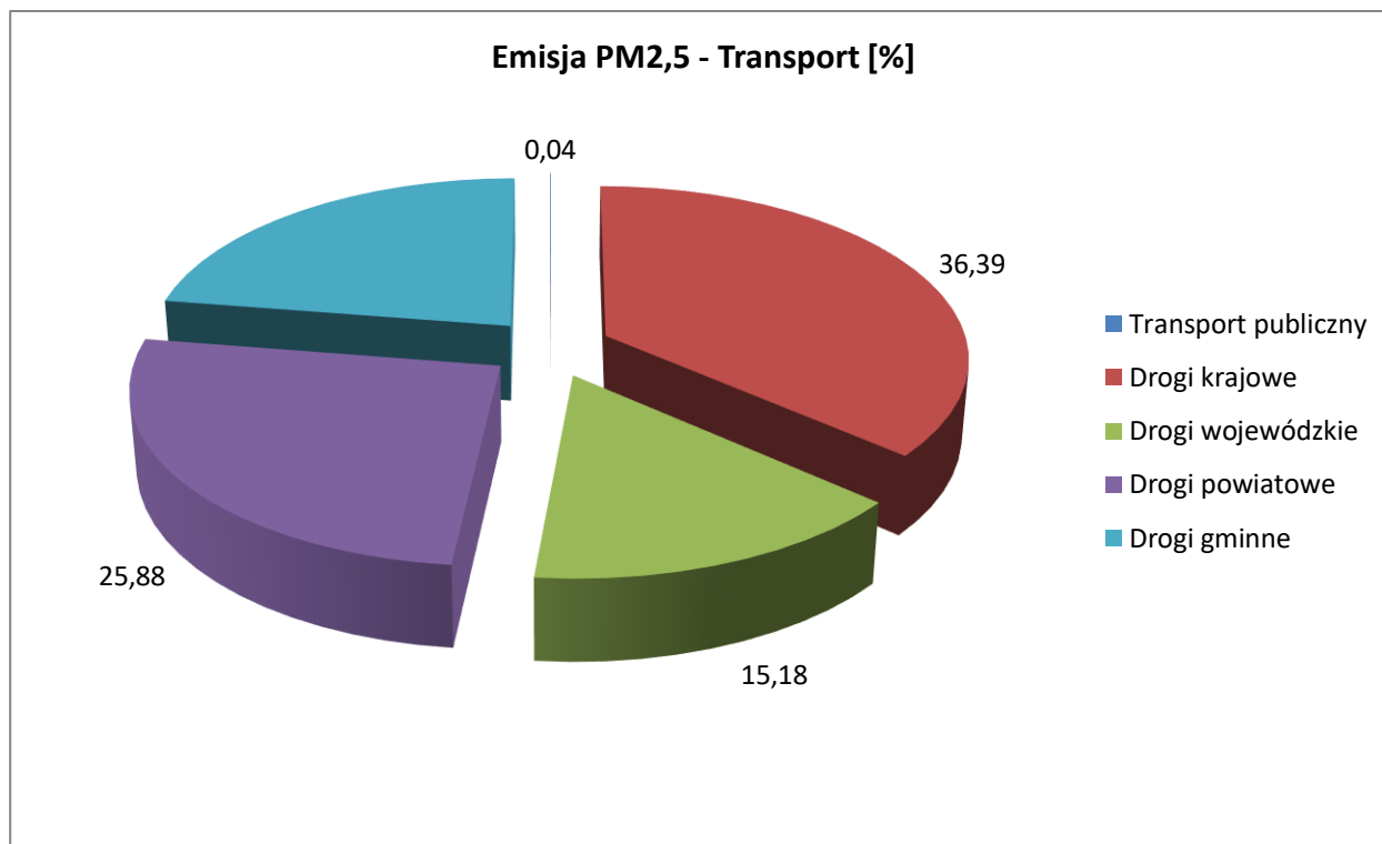
Rysunek 19. Emisja PM2,5 wg. poszczególnych sektorów transportu.
