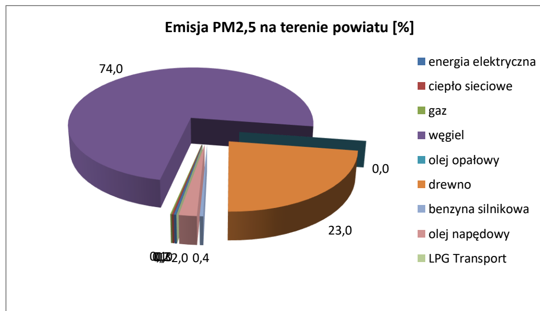
Rysunek 10. Emisja PM2,5 w powiecie wg. rodzajów paliw.
