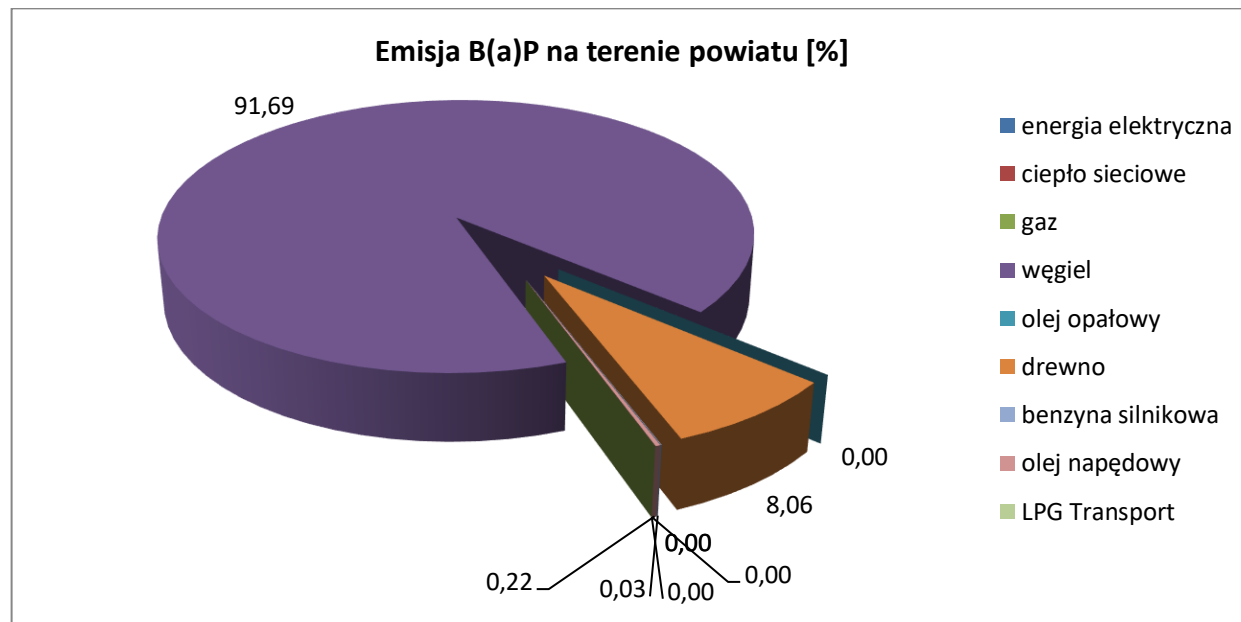
Rysunek 12. Emisja B(a)P w powiecie wg. rodzajów paliw.
