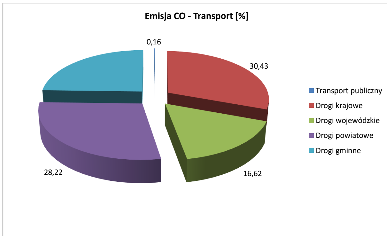
Rysunek 15. Emisja CO wg. poszczególnych sektorów transportu.
