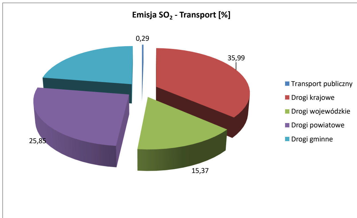
Rysunek 16. Emisja SO 2 wg. poszczególnych sektorów transportu.
