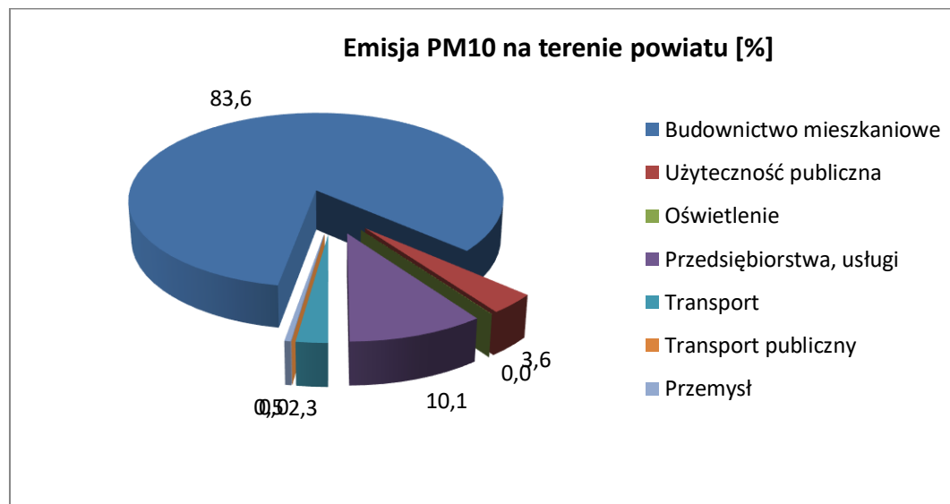
Rysunek 9. Emisja PM10 w powiecie wg. sektorów.
