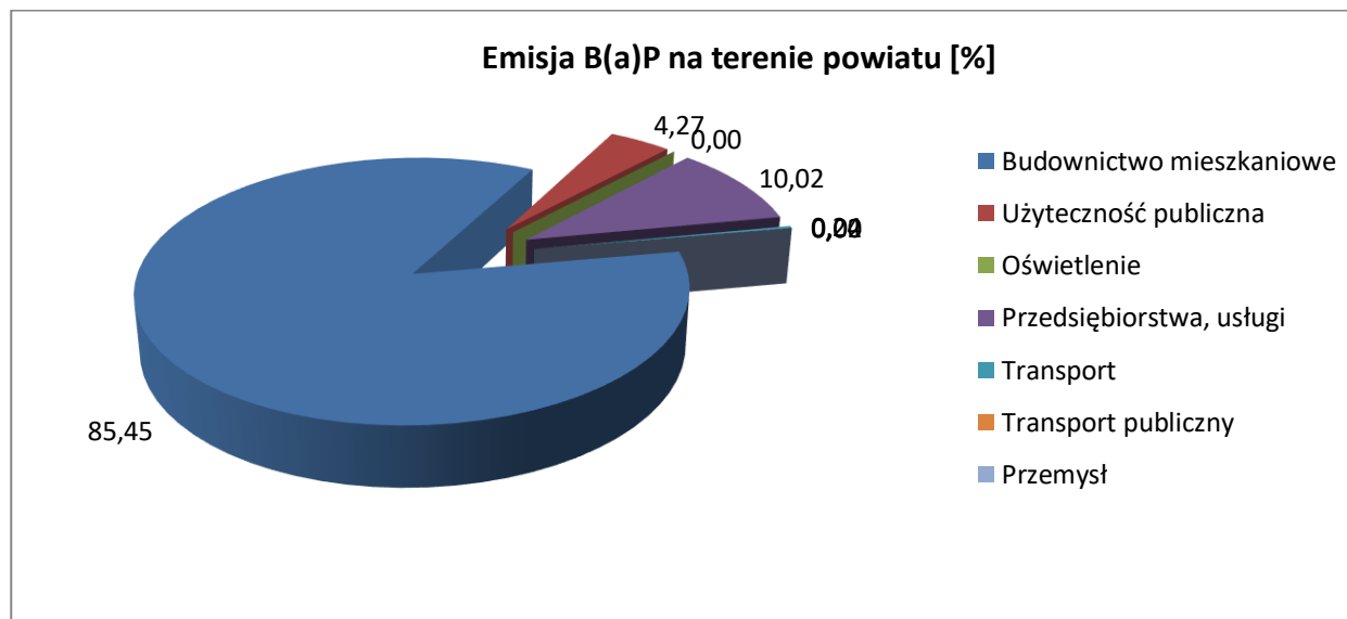
Rysunek 13. Emisja B(a)P w powiecie wg. sektorów.
