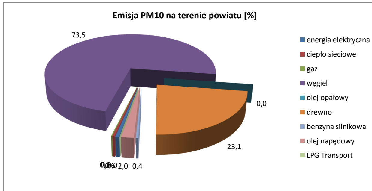
Rysunek 8. Emisja PM10 w powiecie wg. rodzajów paliw.
