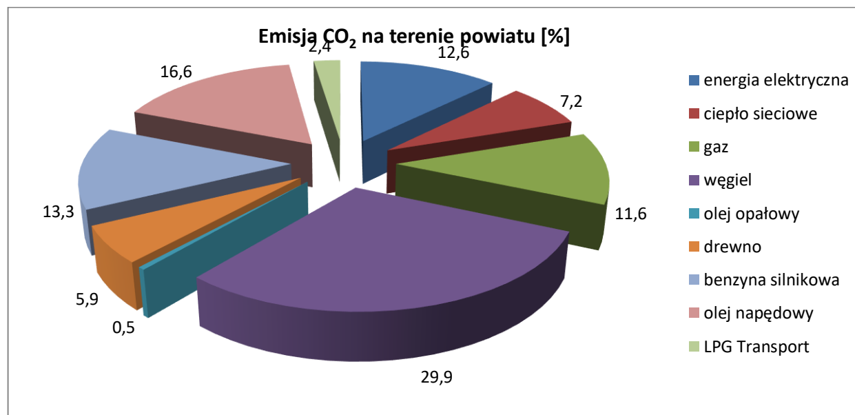
Rysunek 6. Emisja CO 2 w powiecie wg. rodzajów paliw.
