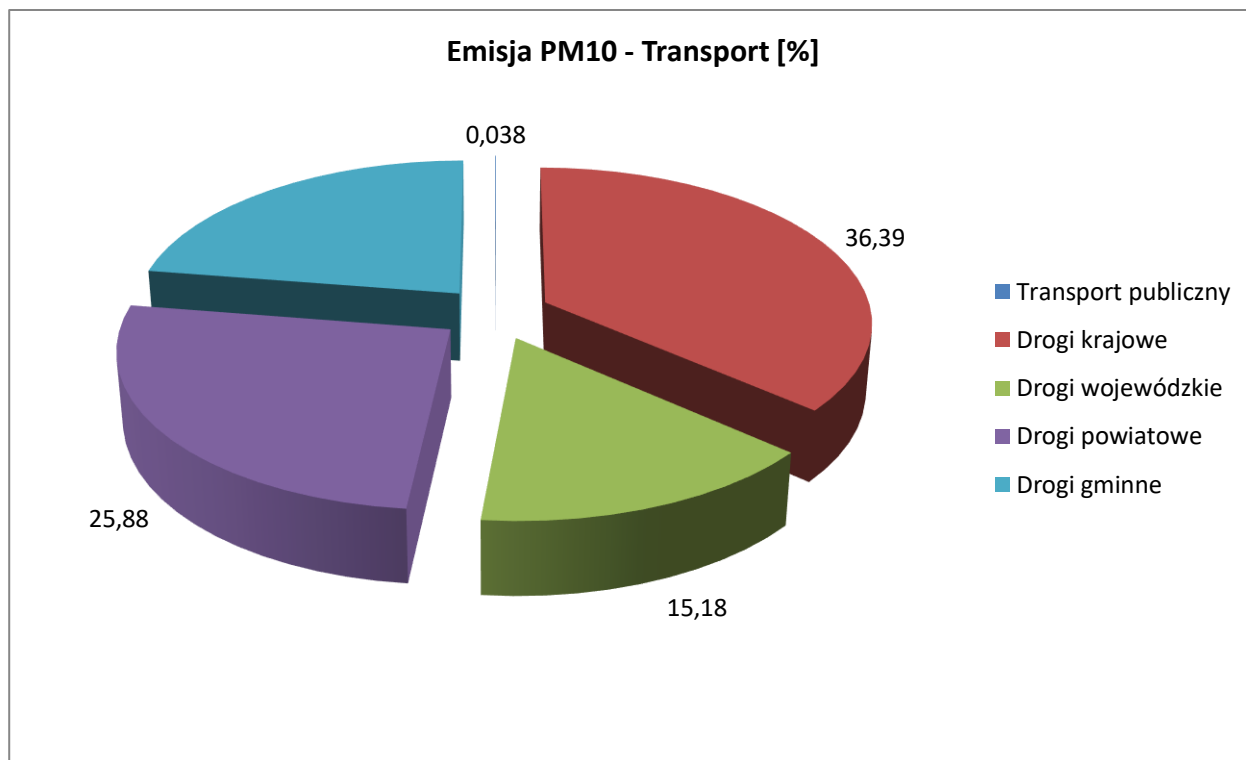
Rysunek 18. Emisja PM10 wg. poszczególnych sektorów transportu.
