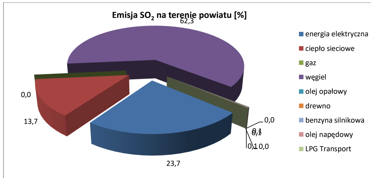
Rysunek 4. Emisja SO 2 w powiecie wg. rodzajów paliw.
