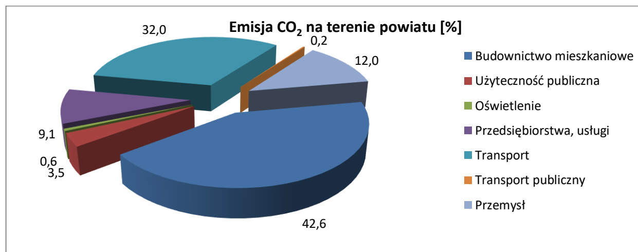
Rysunek 7. Emisja CO 2 w powiecie wg. sektorów.
