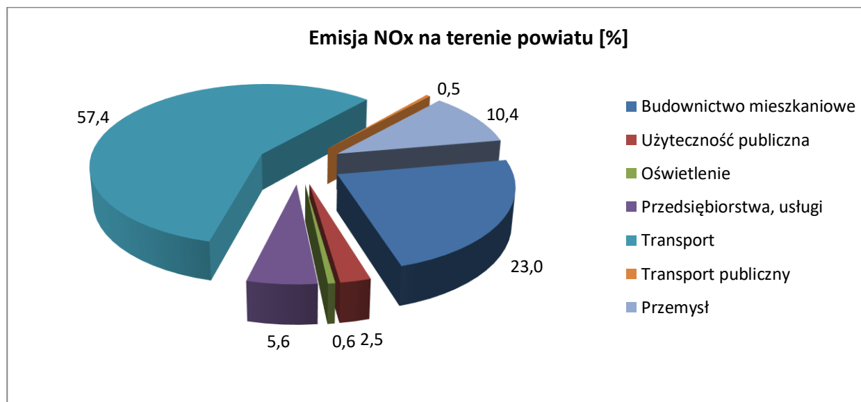
Rysunek 7. Emisja NOx w powiecie wg. sektorów.
