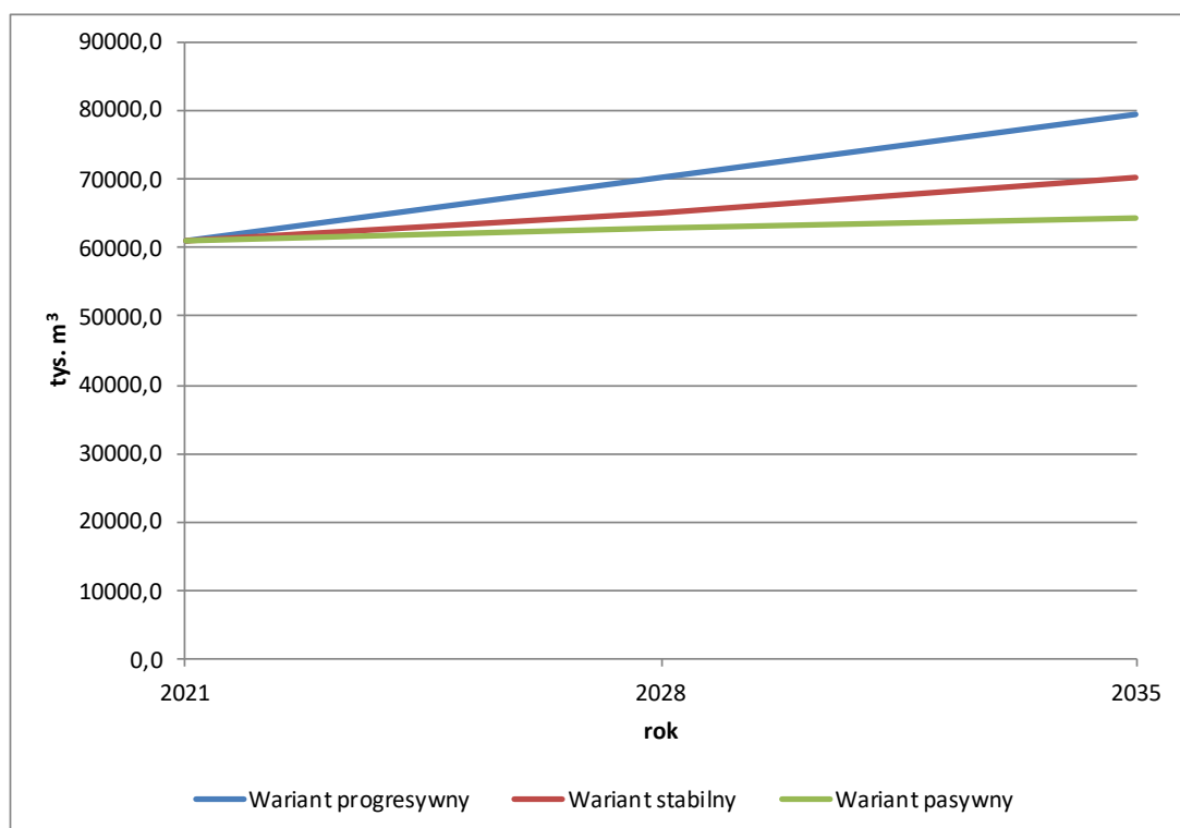
Rysunek 40. Prognozowana zmiana rocznego zużycia paliw gazowych do roku 2035.
